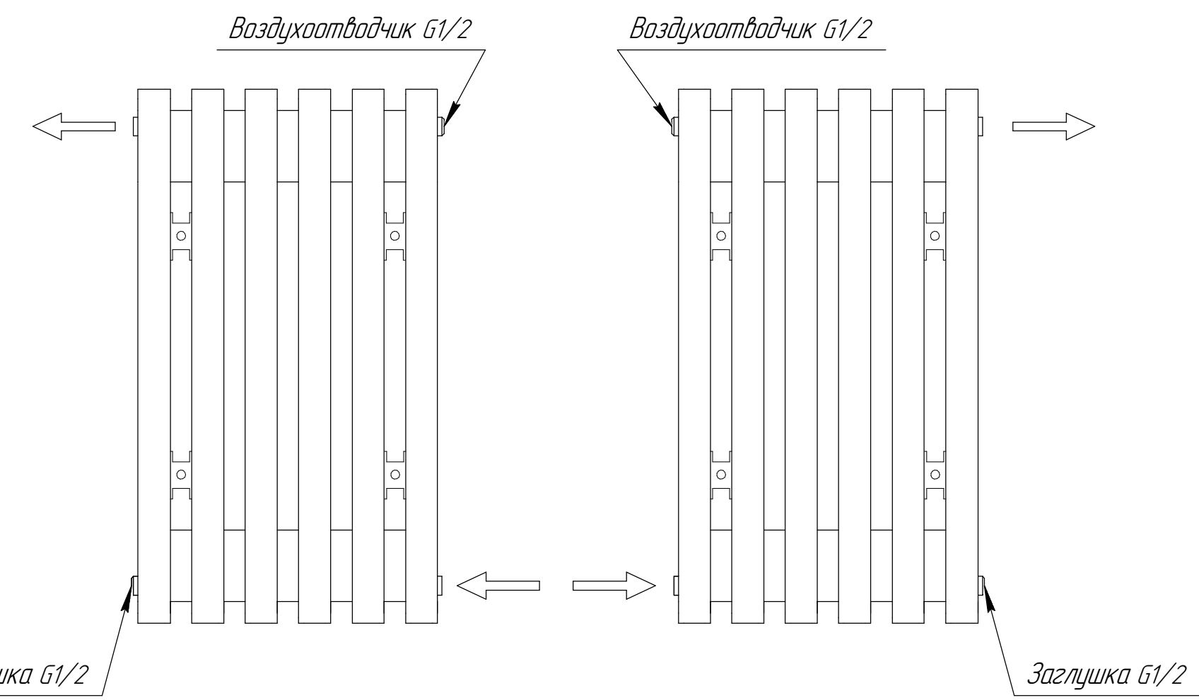
Подключение диагональное
