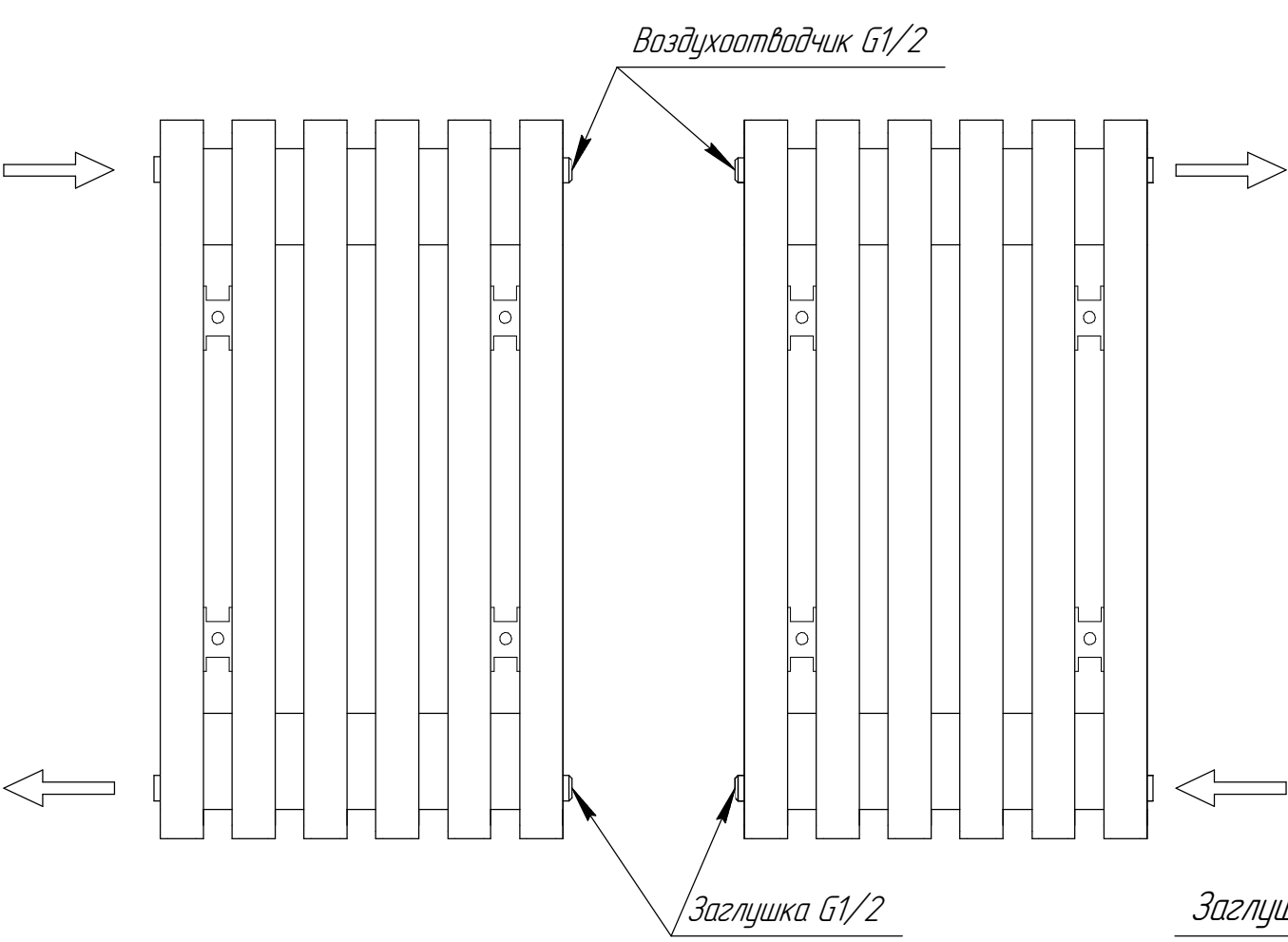
Подключение боковое
