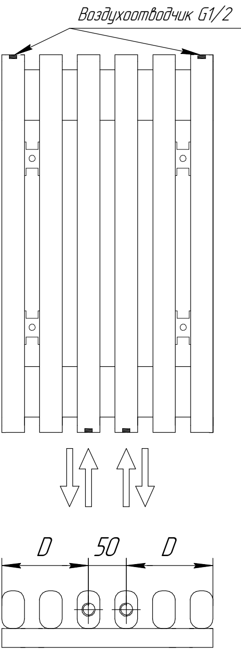
Подключение нижнее "динаклем" 050
