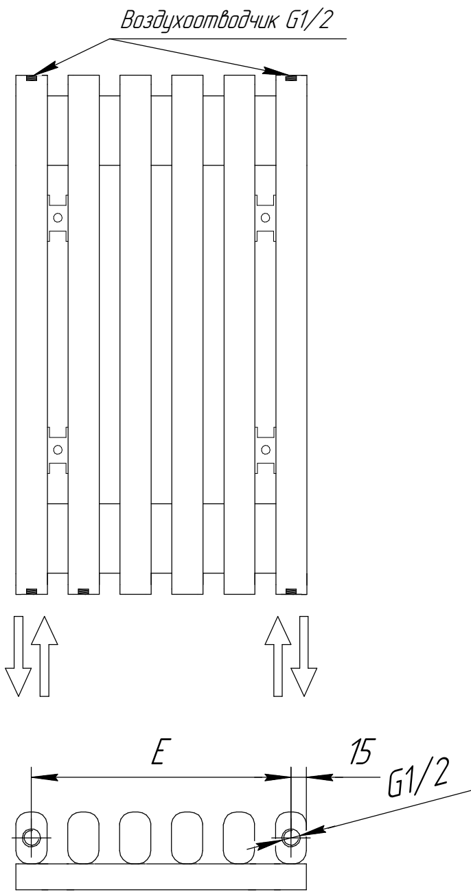
Подключение нижнее разнесенное 117
