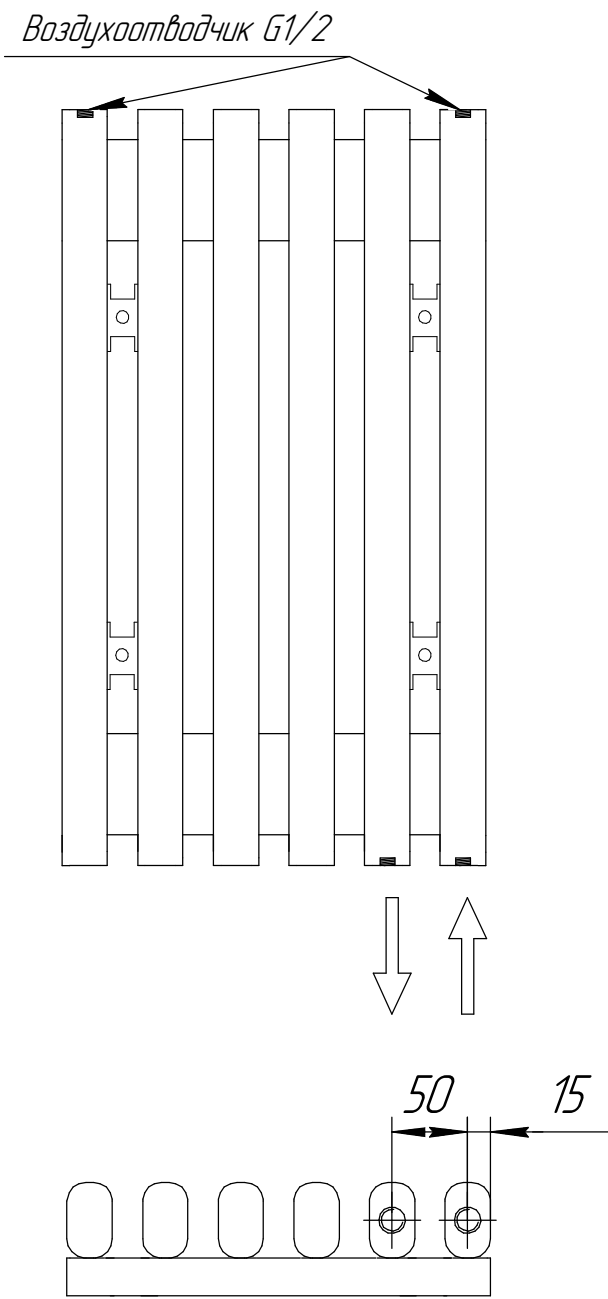
Подключение нижнее "динаклем" 150
